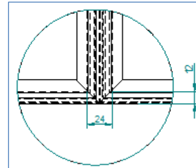
Maß Magnetdichtung
