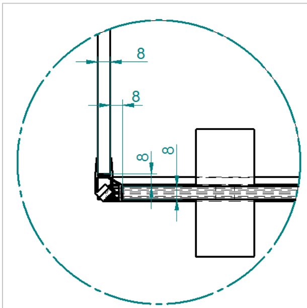
Vermaßung Magnetdichtung
