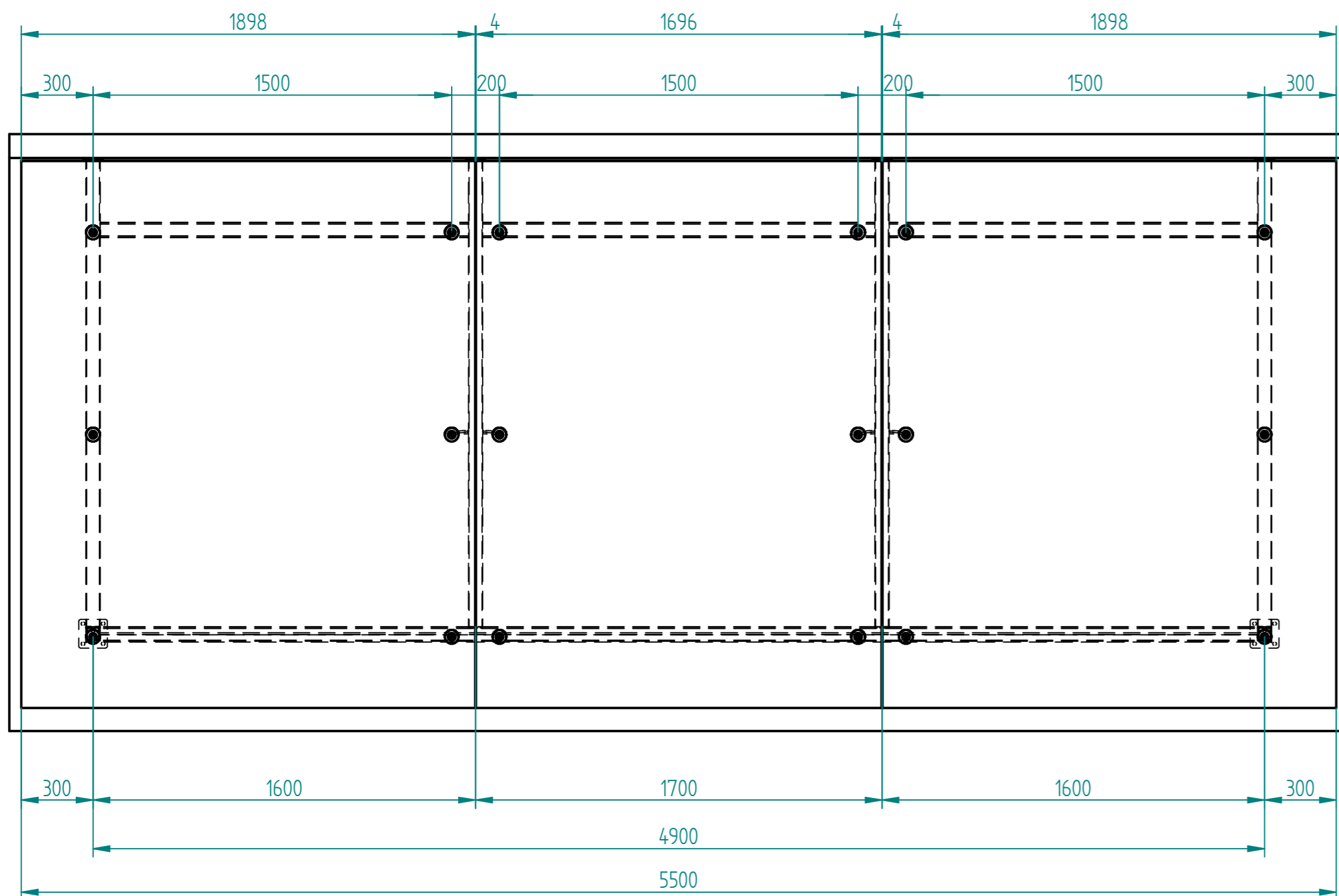
EINZELHEIT B 1:5
