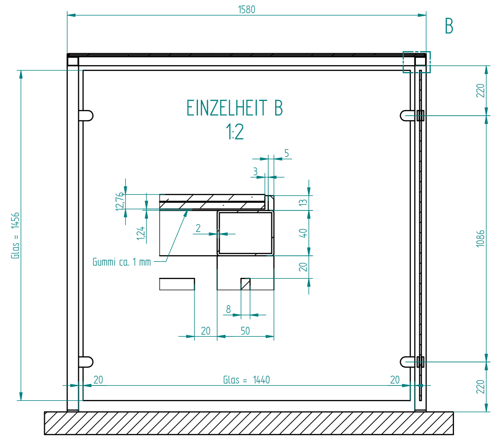
Schnitt A-A
