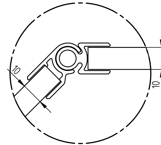
EINZELHEIT A
