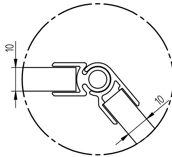
EINZELHEIT A
