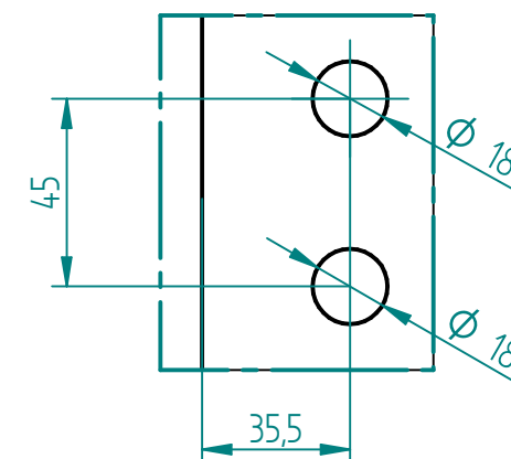
EINZELHEIT A 1:2
