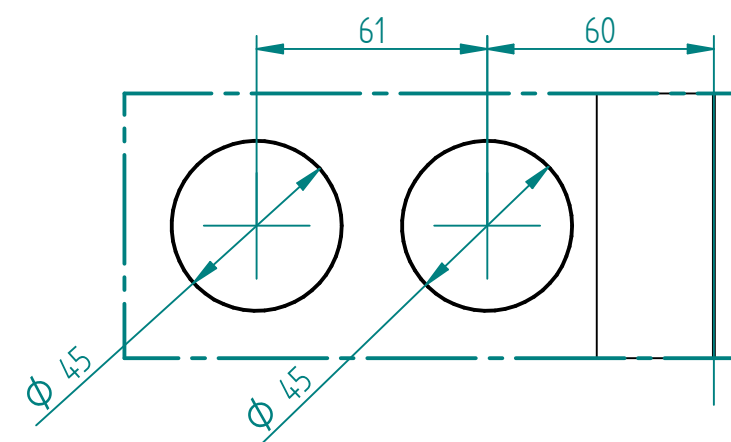
EINZELHEIT B 1:2
